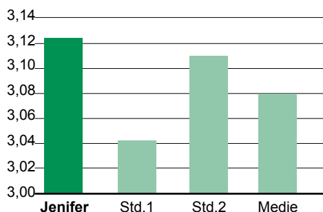
Romania 2010-2012 - medie (13 trials) Productie (t/ha)
